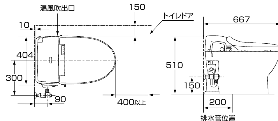
施工完了図 (壁給水タイプの場合)
