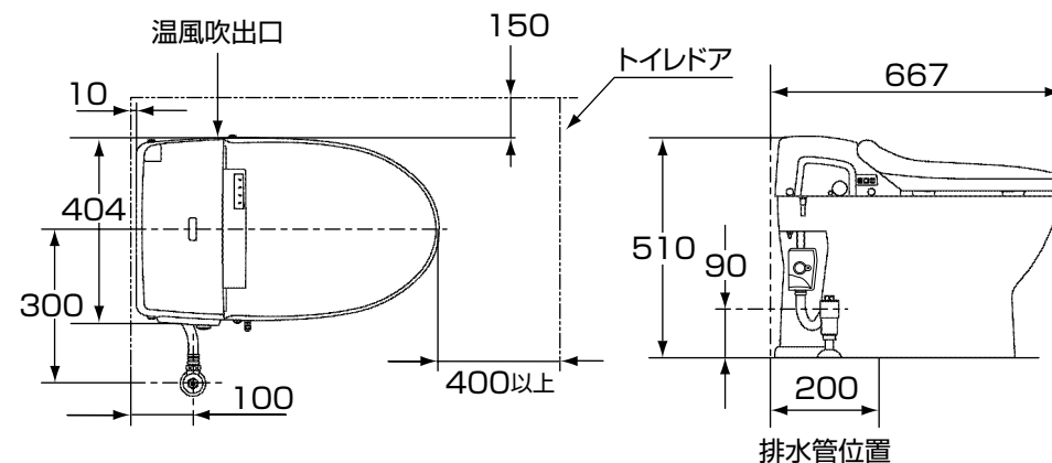
施工完了図 (床給水タイプの場合)
