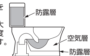
<参考>防露便器、タンクの構造
