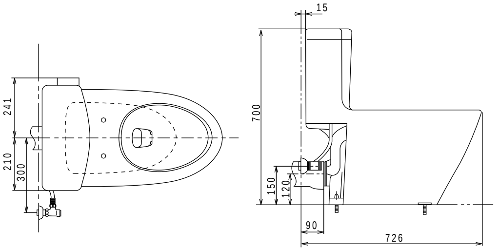
施工完了図（壁給水タイプの場合）
