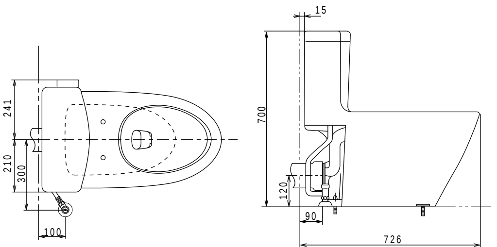
施工完了図（床給水タイプの場合）
