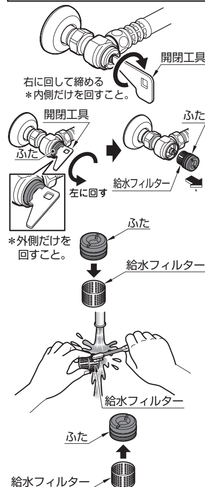
■ 止水栓 (D10094Z)
