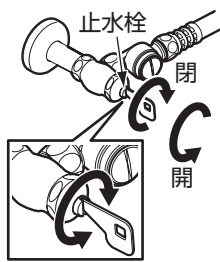
開閉工具 (付属品)
