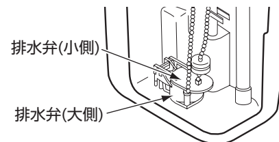
排水弁(小側)
