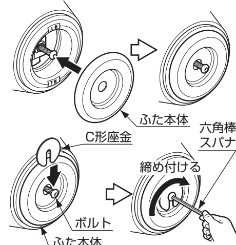
ボルトを自立させる
