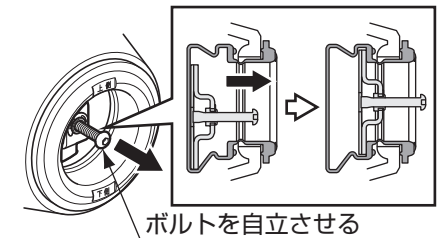
ボルト一体型止め金具
