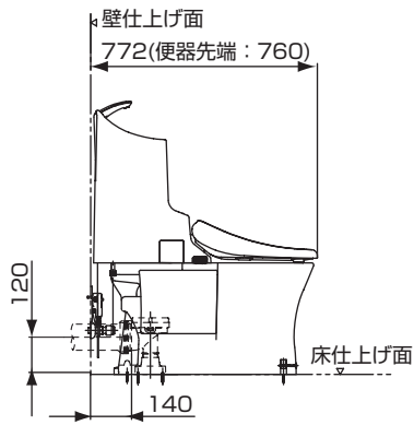
商品セット図 (施工完了図) 床給水タイプ
