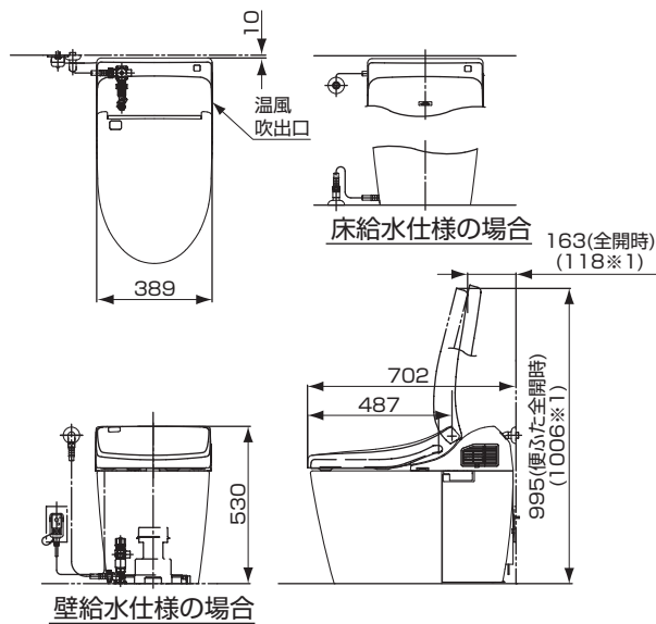
商品セット図 (施工完了図) RHタイプ
