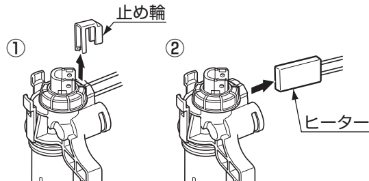
ヒーターの形状が板状の場合
