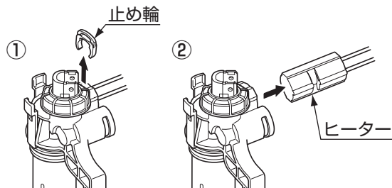
ヒーターの形状が円柱の場合
