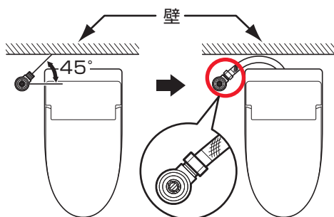
床給水の場合の止水栓取り出し方向
