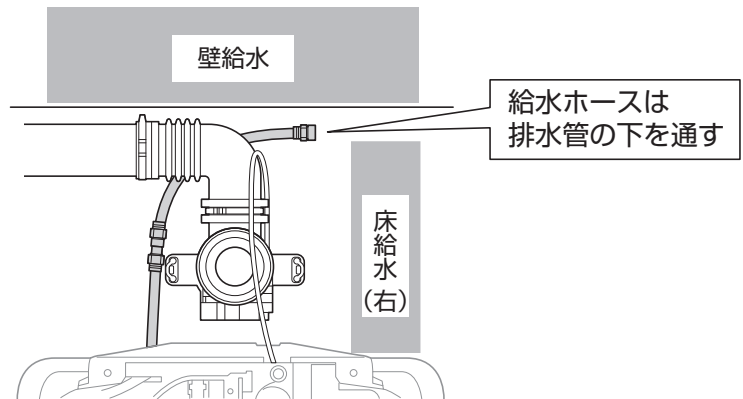
壁給水および床給水（右）の場合
