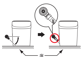
壁給水の場合の止水栓取付方向
