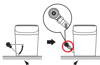
壁給水の場合の止水栓取付方向
