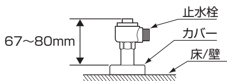
止水栓高さ
