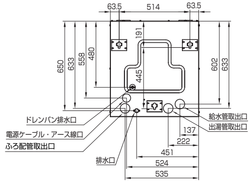
上面透視図
