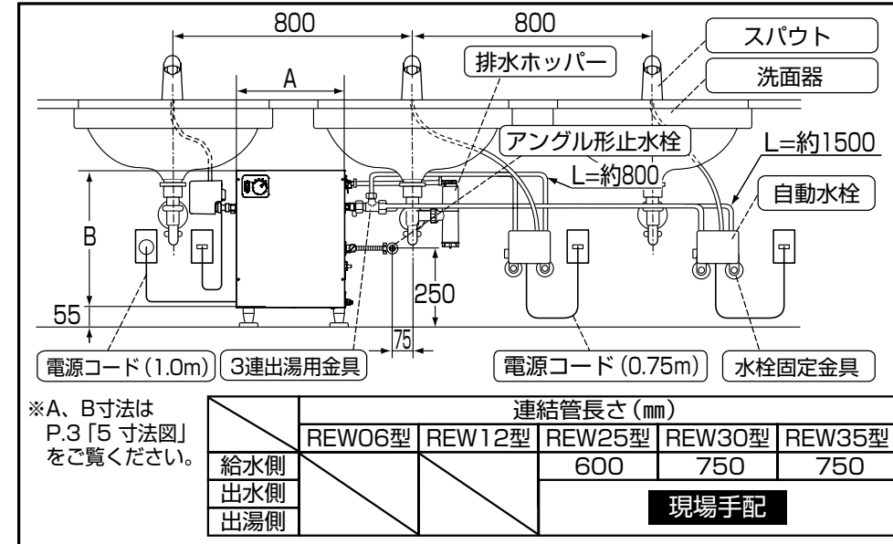
自動水栓 洗面器3連設置例（図はREW35型の例）
