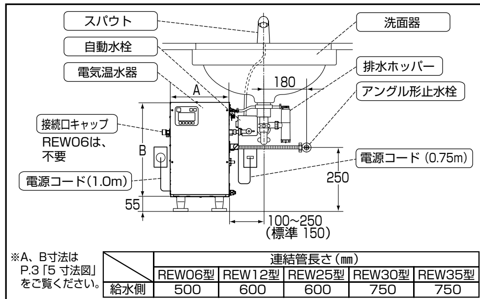
自動水栓 洗面器1連設置例（図はREW12型の例）
