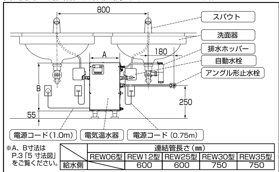
自動水栓 洗面器2連設置例（図はREW12型の例）
