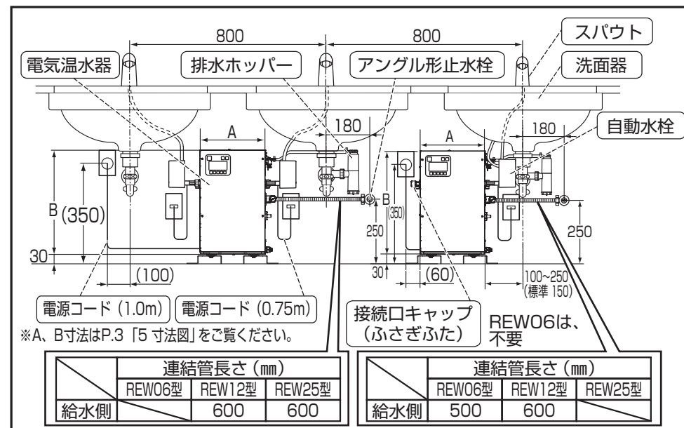
自動水栓 洗面器3連設置例
