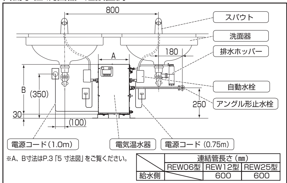
自動水栓 洗面器2連設置例
