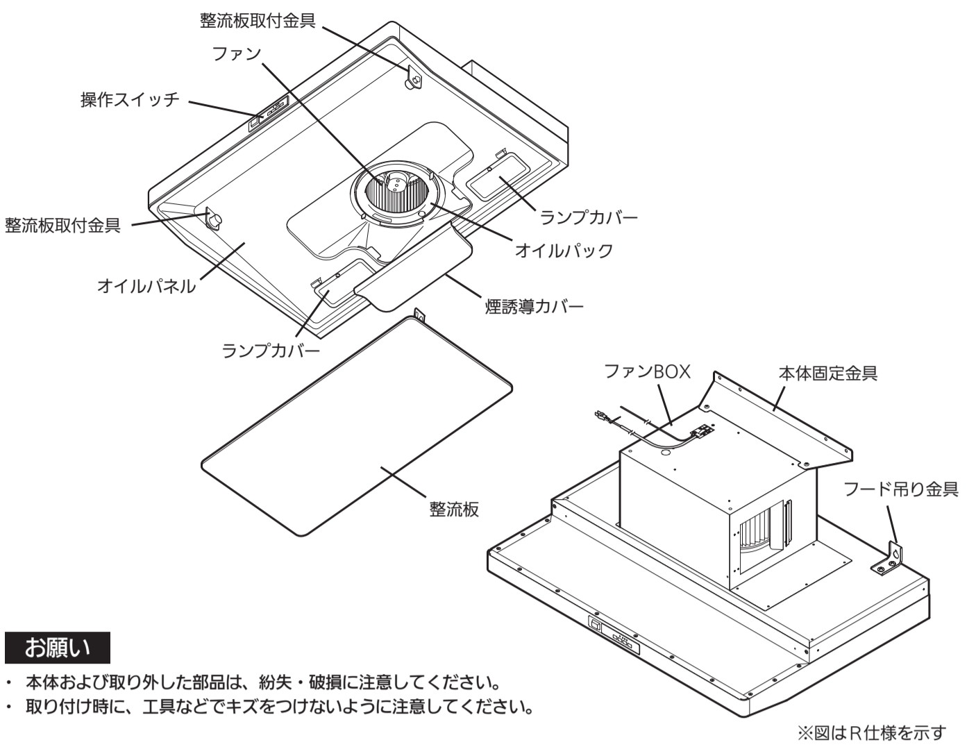
※図はR仕様を示す
