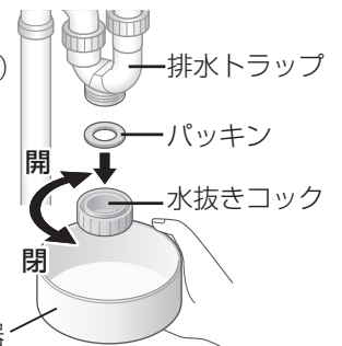
水受け容器
