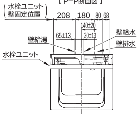
【P-P断面図】
