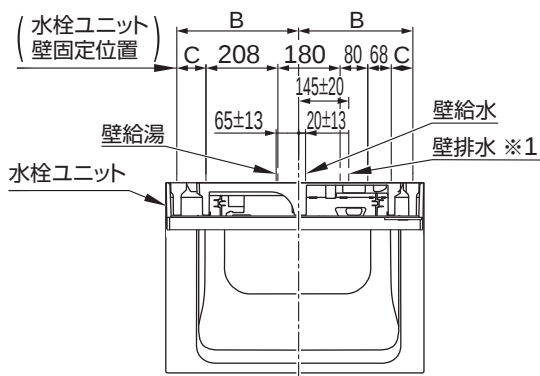
【P-P断面図】
