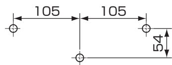
壁取付ねじ位置
